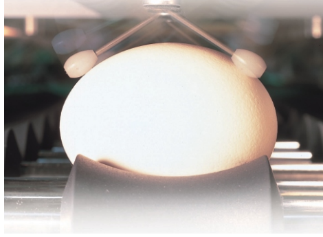
Otomatik Çatlak Dedektörü (OP)
